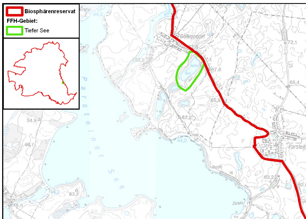
Abb. 1: Lage des FFH-Gebiets Nr. 422 : Tiefer See
