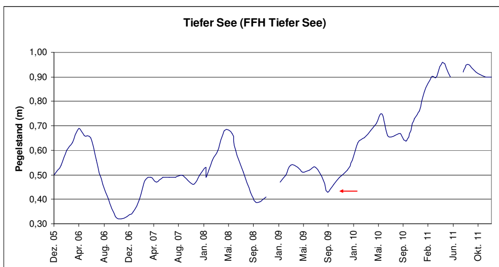
Abb. 5: Pegeldata des Tiefen Sees für den Zeitraum 12/2005 – 12/2011
