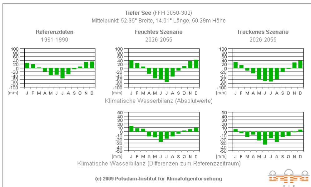
Abb. 4: Klimatische Wasserbilanz nach PIK (2009)
