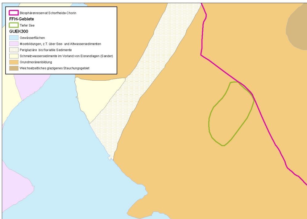
Abb. 2: Geologische Übersichtskarte (GUEK300)
