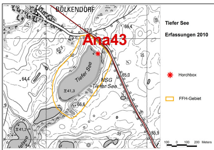
Abb. 11: Horchboxstandort im FFH-Gebiet Tiefer See (vgl. Tab. 12)
