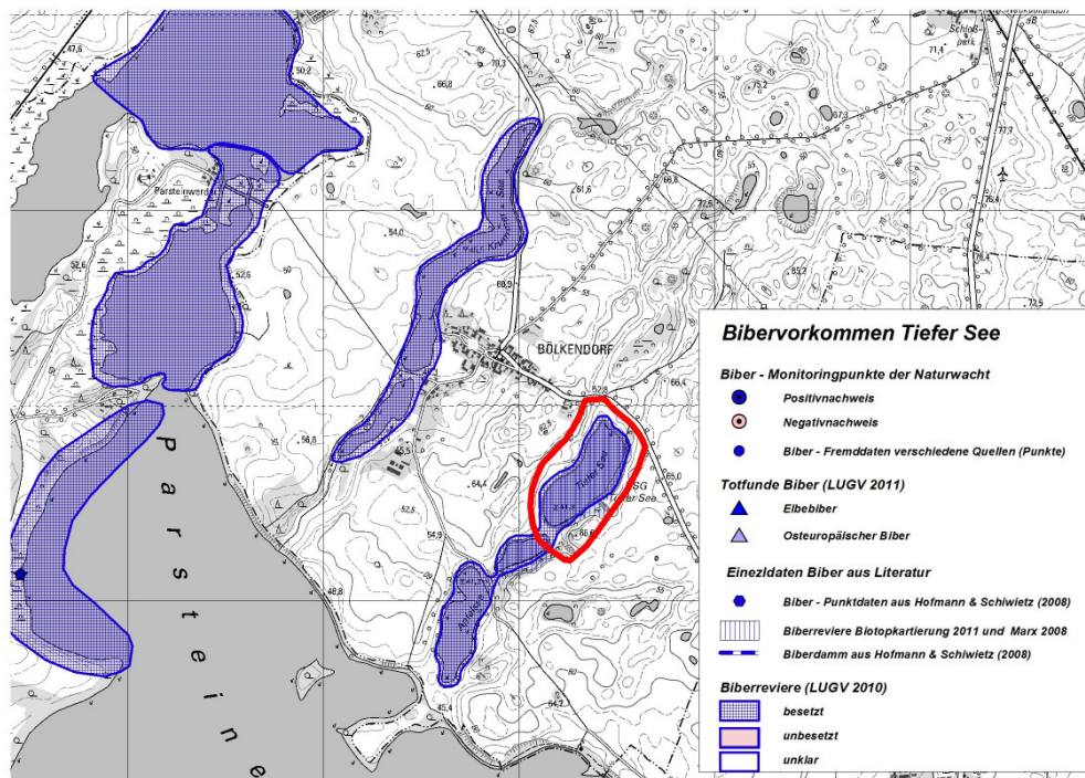
Abb. 10: Verbreitung des Bibers
