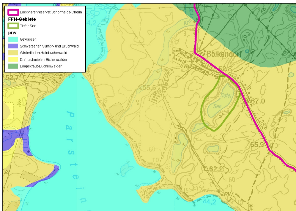
Abb. 6: PNV (HOFMANN & POMMER 2005)
