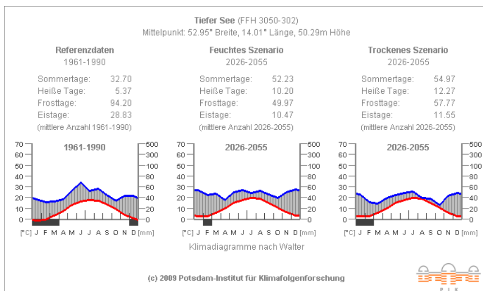
Abb. 3: Klimaszenarien nach PIK (2009)
